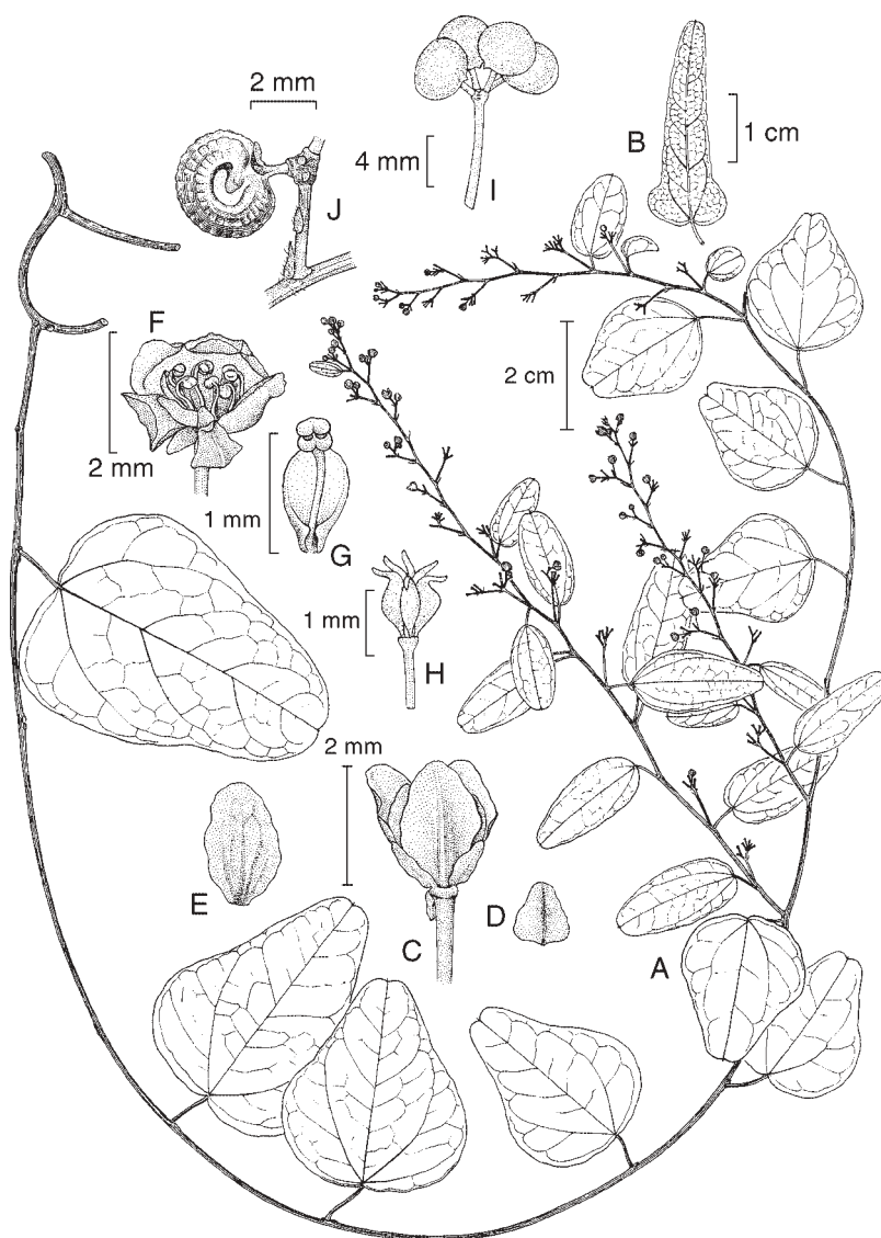
Cocculus diversifolius DC. A. rama con hojas e inflorescencias masculinas; B. hoja hastada; C. disposición del perianto; D. sépalo intermedio; E. sépalo interno; F. flor masculina; G. pétalo y estambre; H. gineceo; I. frutos; J. hueso. Ilustrado por E. Saavedra y reproducido con algunas modificaciones del fascículo 87 de la Flora de Veracruz.
